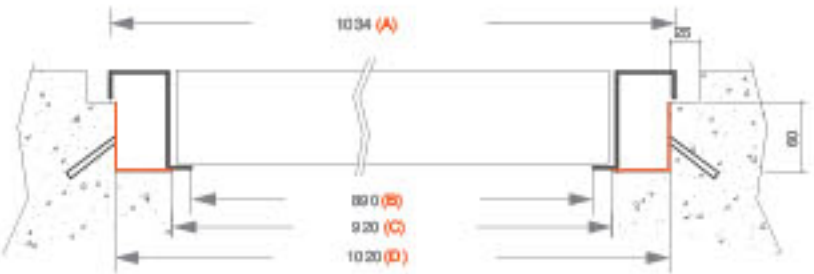
Sezione orizzontale Horizontal section Sección horizontal
