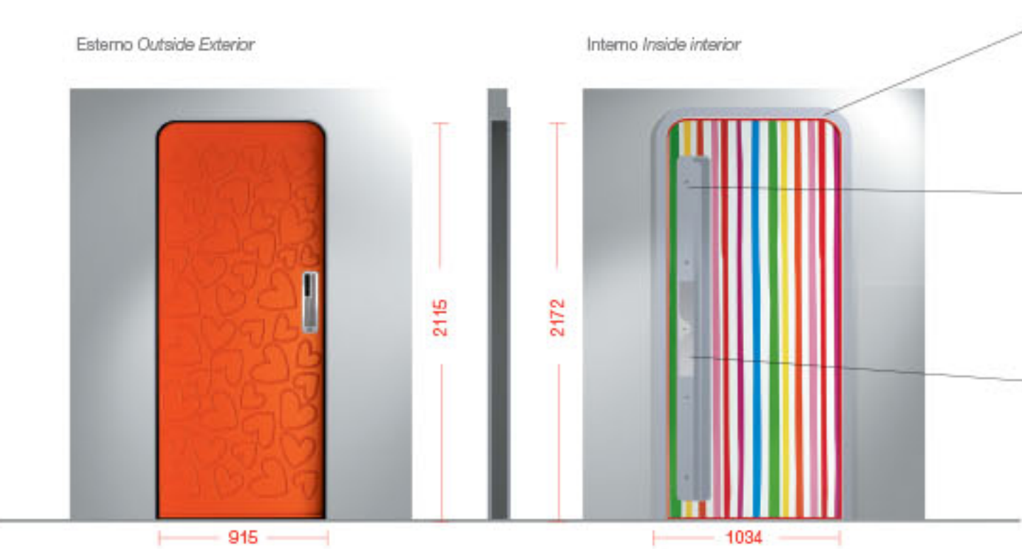
Anta spessore 80 mm Door thickness 80 mm Espesor de la Hoja 80 mm
